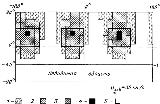
Рис. 36. Карта распределения локальных эквивалентных ширин (модель 1): 1 — 0,03–0,08 А; 2 — 0,08–0,13 А; 3 — 0,13–0,18 А; 4 — 0,18–0,23 А; 5 — контуры исходного распределения
