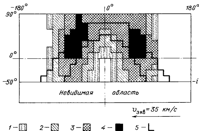
Рис. 38. Карта распределения локальных эквивалентных ширин (модель 2): 1 - 0,02–0,05 Å; 2 - 0,05–0,08 Å; 3 - 0,08–0,011 Å; 4 - 0,11–0,14 Å; 5 - контуры исходного распределения
