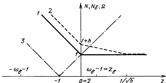
Рис. 11. Графики функционалов: 1 — N(z) = \|Az - \bar{u}\|^2 ; 2 — N_\delta(z) = \|A_h z - \bar{u}\|^2 ; 3 — \Omega(z)
