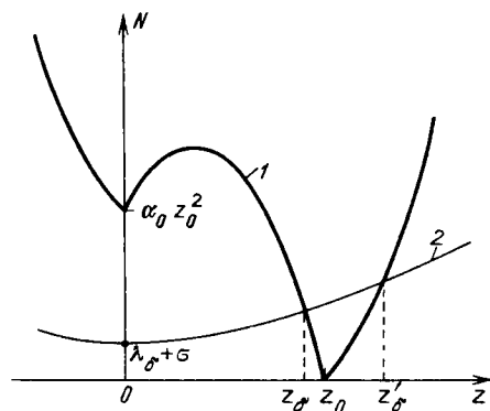
Рис. 5. Иллюстрация к примеру 1: 1 — невязка N(z) = \|Az - \bar{u}\|^2 ; 2 — \pi(z) = (\lambda_{\delta} + \sigma + h|z|)^2
