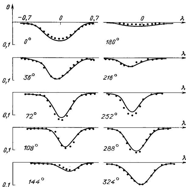
Рис. 39. Профили линий: модельные ····; вычисленные —. Среднеквадратичная погрешность - - 0,008
