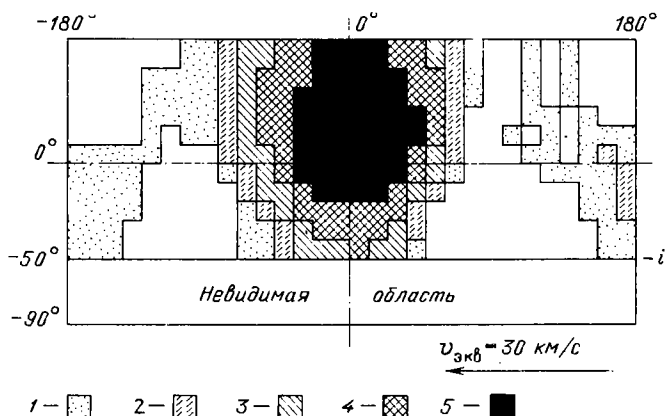
Рис. 42. HD 112412, \lambda 4129 Å Eu II. Карта распределения локальных эквивалентных шириин: 1 — 0,35—0,70 Å; 2 — 0,70—0,105 Å; 3 — 0,105—0,140 Å; 4 — 0,140—0,175 Å; 5 — 0,175—0,210 Å
