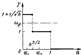
Рис. 13. График функции \gamma(\alpha)
