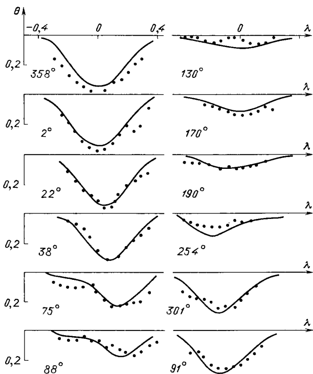
Рис. 43. HD 112412, \lambda 4129 Å Eu II. Профили линий: наблюдаемые — вычисленные —
